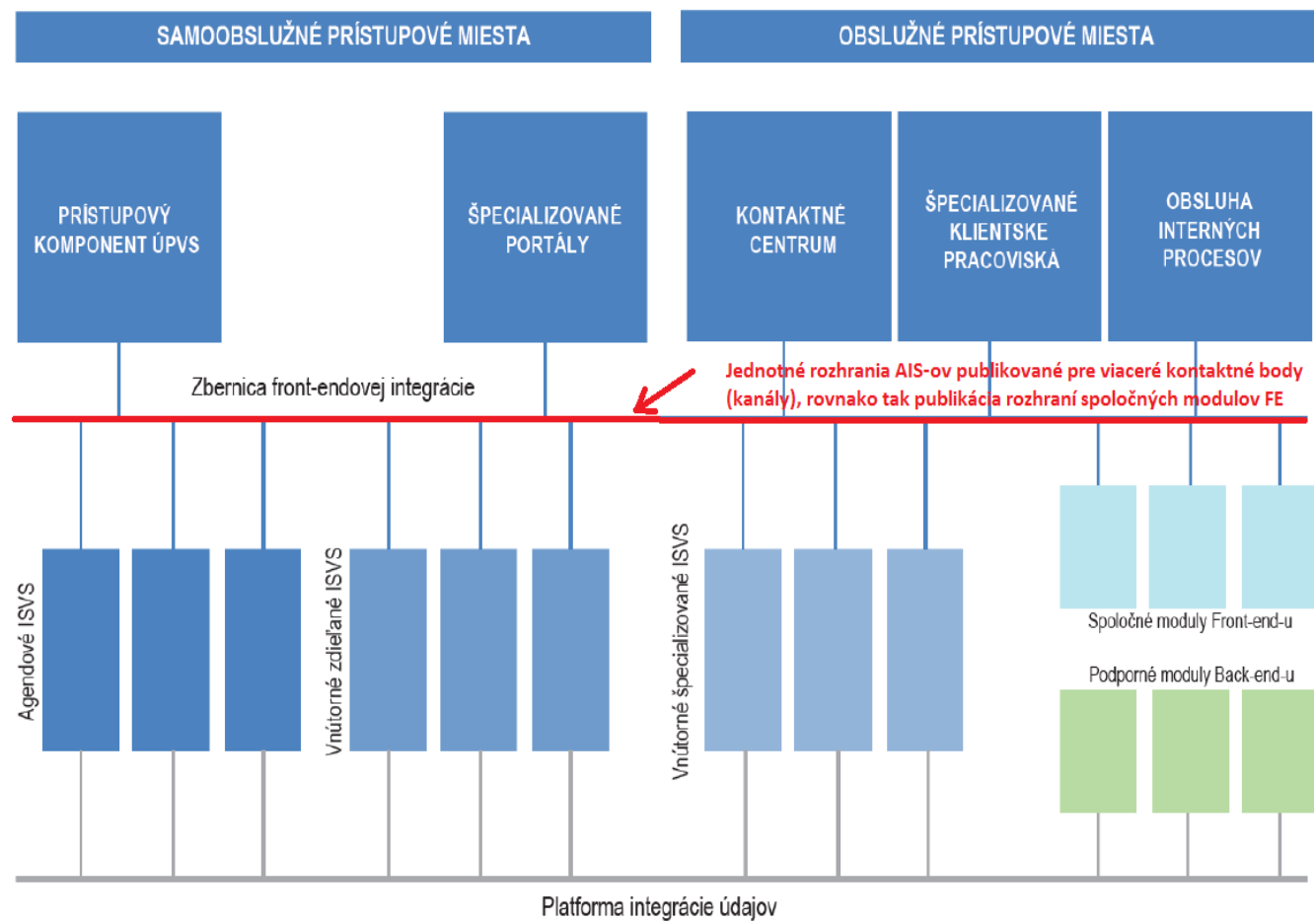
Obrázok 4: Schéma referenčnej architektúry IIS VS.
