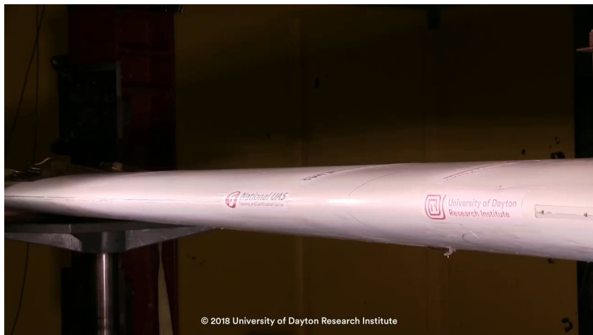
Testovanie zrážky s dronom (University of Dayton)
