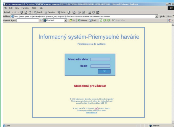
HTML klient
